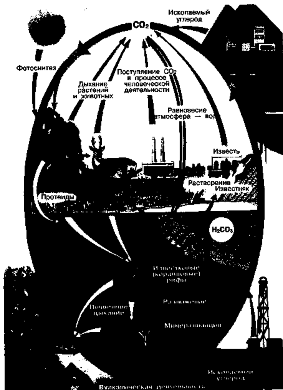
Рис. 107. Круговорот углерода
