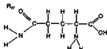
Глутамин (гln)
